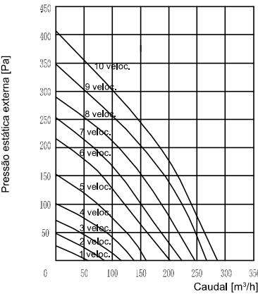
VMC EX 250
